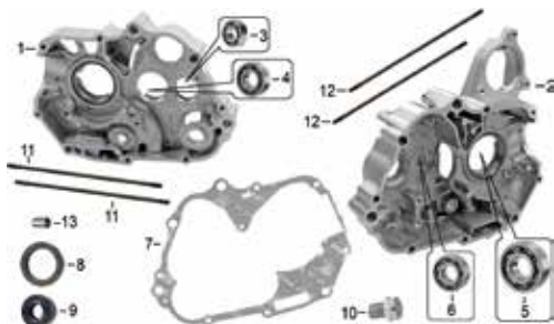
CÁRTER E-7
