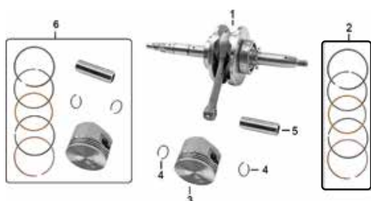
CIGÜEÑAL E-8
