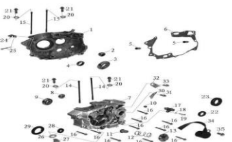
FIG.8 CARCASAS MOTOR
