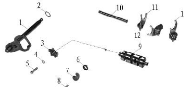
FIG11 EJE CAMBIOS ,SELECTOR,HORQUILLAS
