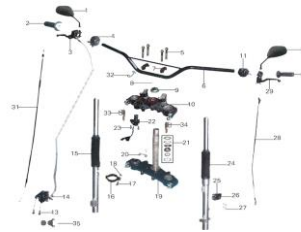
FIG 14 MANUBRIO,COMANDOS,ESPIGO,TELESCOPICOS
