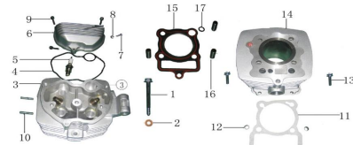
FIG.1 TAPA CULATA,CULATA ,CILINDRO
