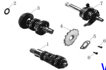
FIG.10 EJE PRIMARIO,SECUNDARIO, ARRANQUE
