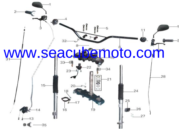
FIG.14 MANUBRIO,COMANDOS,ESPEJOS,MENSULA,ESPIGO DIRECCION,TELESCOPICOS
