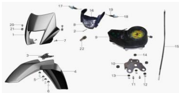
FIG.13 FAROLA ,CUBIERTA FAROLA,VELOCIMETRO
