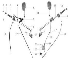
FIG.17 ESPEJOS,MANUBRIOS,COMANDOS,MANILARES
