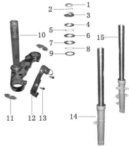
FIG.19ESPIGO,MENSULA,TELESCOPICOS,TELESCOPICO
