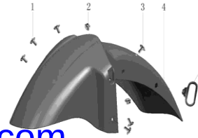
FIG.21 GUARDABARRO DELANTERO
