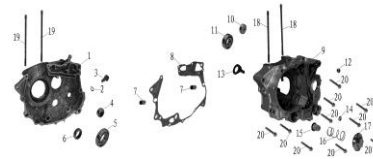
FIG.12 CARCAZAS MOTOR
