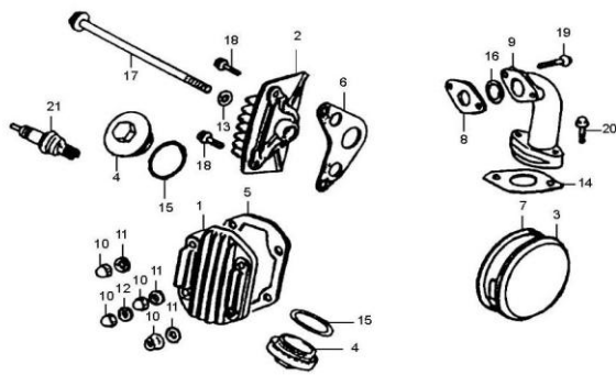
FIG.5 STATOR,TAPA VOLANTE,TAPA PINON DE SALIDA
