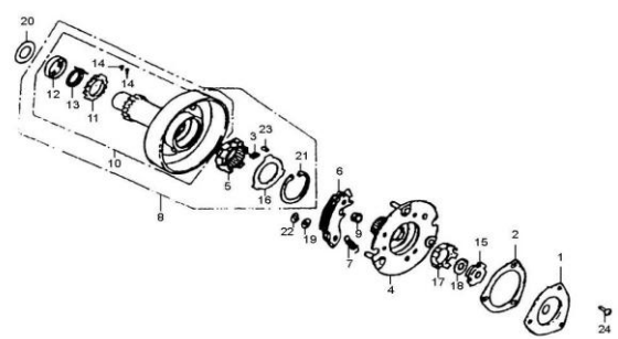
FIG.8 EMBRAGUE PRIMARIO
