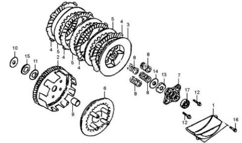
FIG.9 CONJUNTO EMBRAGUE SECUNDARIO
