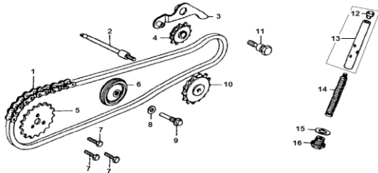
FIG.4 CADENILLA DE DISTRIBUCION,TENSOR ,GUIA
