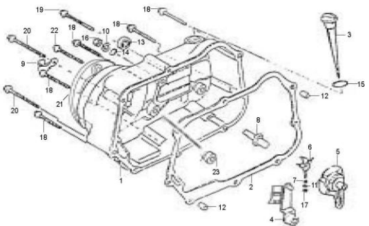
FIG.7 CARCAZA EMBRAGUE
