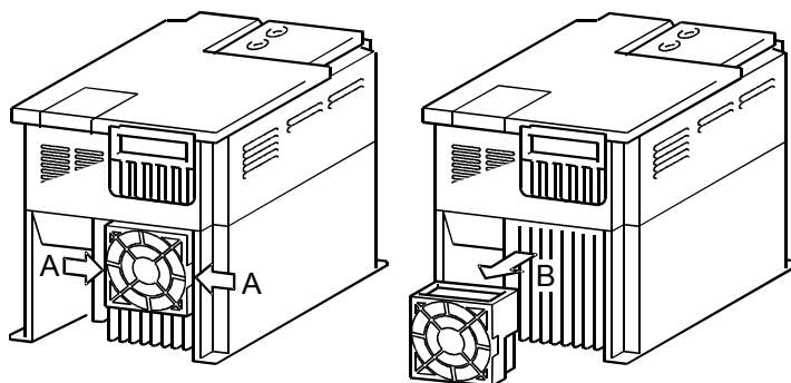
风扇接口
