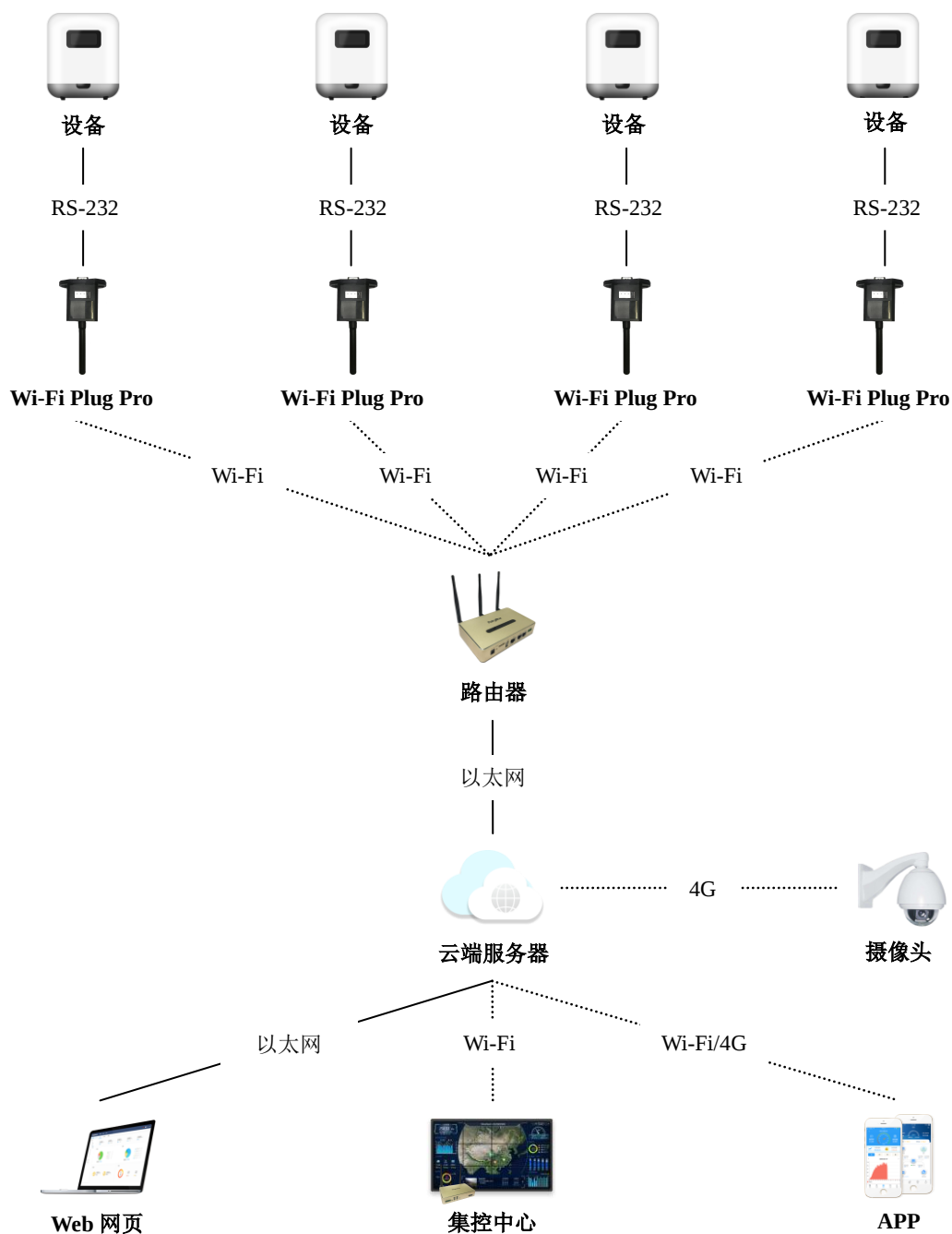
Wi-Fi Plug Pro-03 产品典型组网方案
