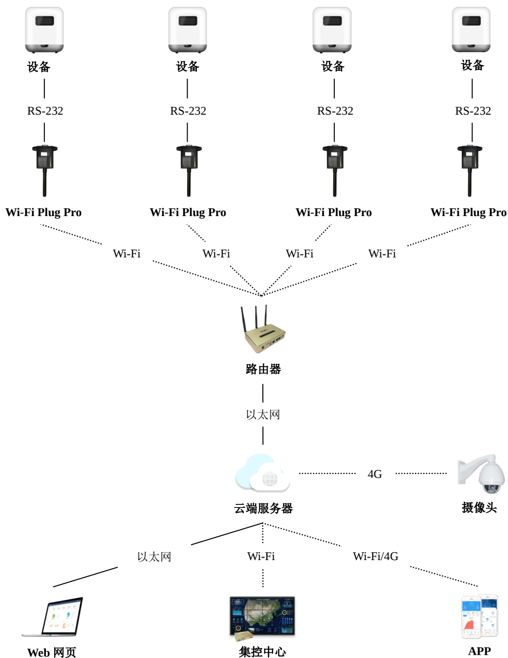
Wi-Fi Plug Pro-05 产品典型组网方案
