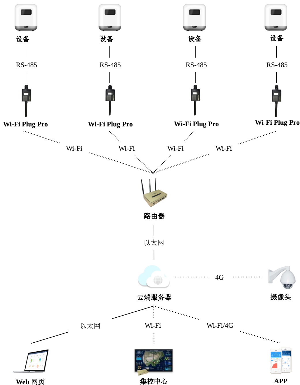
Wi-Fi Plug Pro-02 产品典型组网方案
