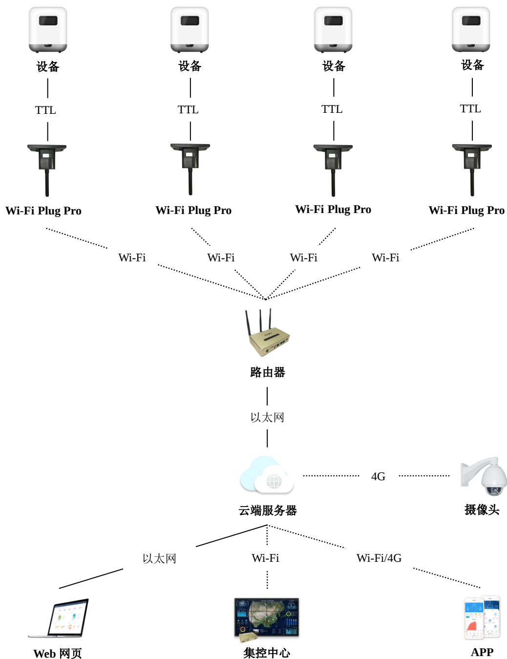
Wi-Fi Plug Pro-01 产品典型组网方案
