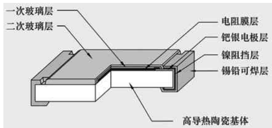
图1 片式厚膜固定电阻器结构图
