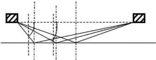
图 5 印刷过程网版形变示意图
