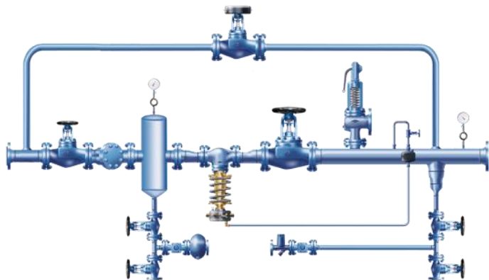
PREsys® 减压系统
