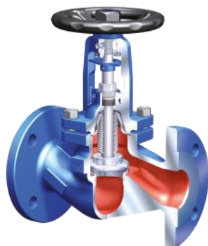
截断阀系列
