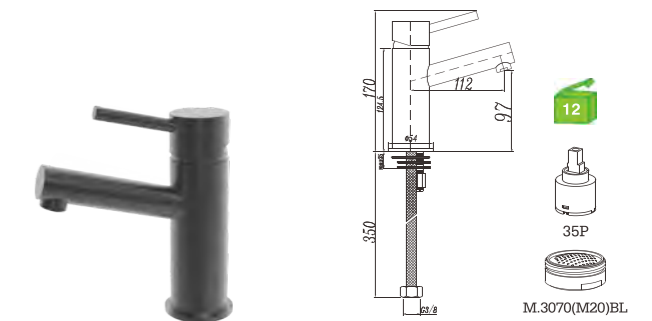
E34GP1BL-1 Monocomando lavatório Basin mixer Monomando lavabo C/bicha certificada S/VÁLVULA
