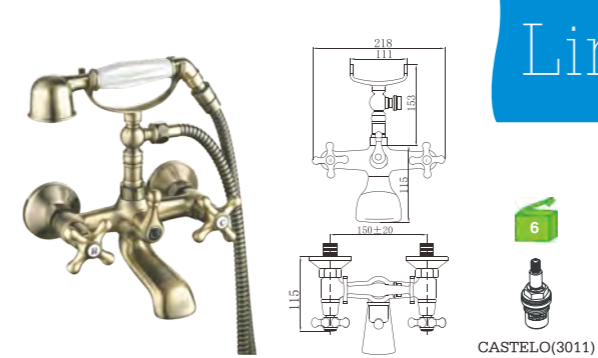
H15T2BR Misturadora banheira Bath/shower mixer Monobloc baño C/CHUVEIRO---888BR BICHA ---2030BR(1.7M) SUPORTE ---MH(BR)
