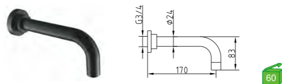
3067BL Bica Caño
