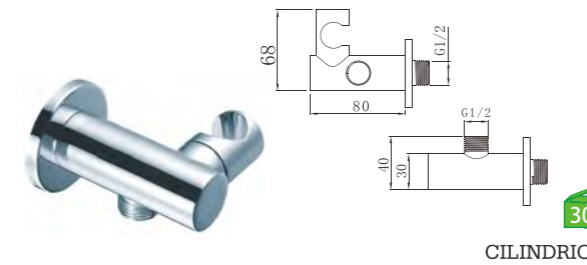
3092 Tomada de água com suporte Toma de água com suporte
