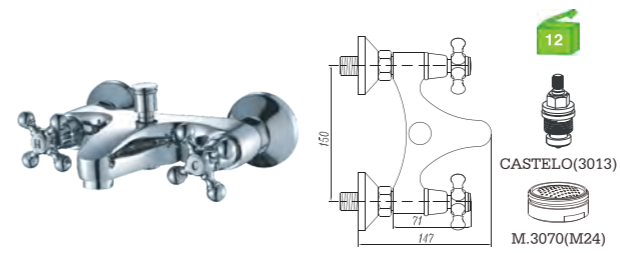
H11T2C Misturadora banheira Bath/shower mixer Monobloc baño C/CHUVEIRO---168 BICHA ---2031(1.7M) SUPORTE ---JH
