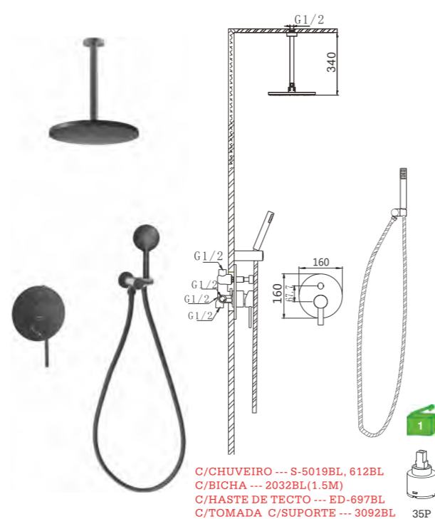
D26FK45BL Conj.Monocomando embutido 2 vias para duche Built-in shower mixer Conj.Monomando empotrado 2 vias para ducha
