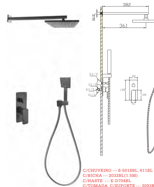
D21RP47BL Conj.Monocomando embutido 2 vias para duche Built-in shower mixer Conj.Monomando empotrado 2 vias para ducha
