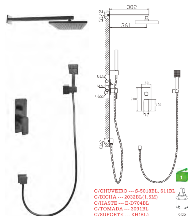
D21RP44BL Conj.Monocomando embutido 2 vias para duche Built-in shower mixer Conj.Monomando empotrado 2 vias para ducha
