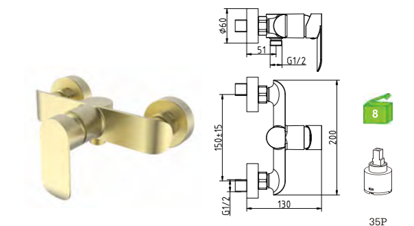
A60UP3LG Monocomando duche Shower mixer Monomando ducha C/CHUVEIRO---190LG BICHA ---2030LG(1.5M) SUPORTE ---PH(LG)
