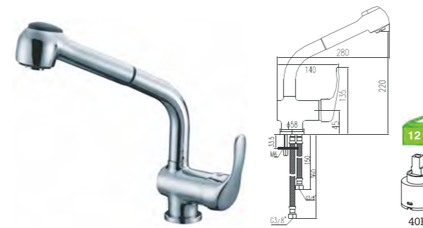
R26M17C C/Bicha Certificada Monocomando lava-loiça com chuveiro Kitchen mixer with pull out shower Monomando fregadero extraible C/CHUVEIRO ---172 BICHA ---2028(1.5M)
