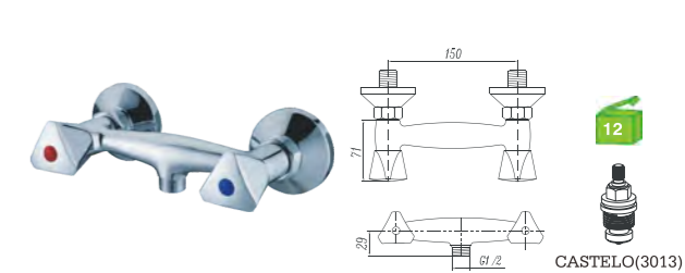
H11033C Misturadora duche Shower mixer Monobloc ducha C/CHUVEIRO---168 BICHA ---2031(1.7M) SUPORTE ---JH
