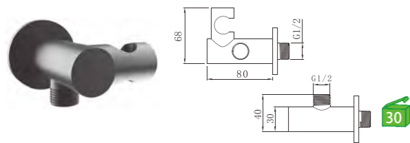
3092BL Tomada de água com suporte Toma de água com suporte
