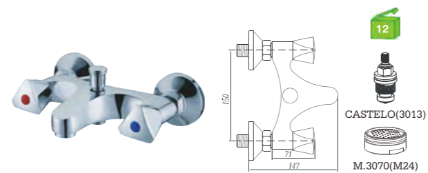
H11032C Misturadora banheira Bath/shower mixer Monobloc baño C/CHUVEIRO---168 BICHA ---2031(1.7M) SUPORTE ---JH
