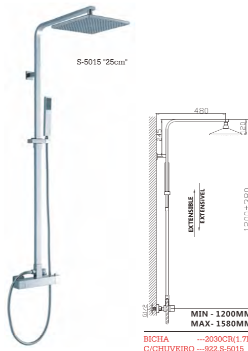
C54KB13C Conj. De duche termostática com torneira Thermostatic shower column with faucet Conj. De ducha termostatico con grifería
