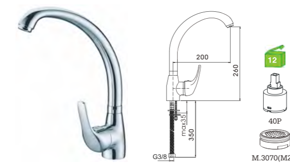
R26M18C C/Bicha Certificada Monocomando lava-loiça à banca bica alta Kitchen mixer Monomando fregadero (caño tubular) BICA ---3064
