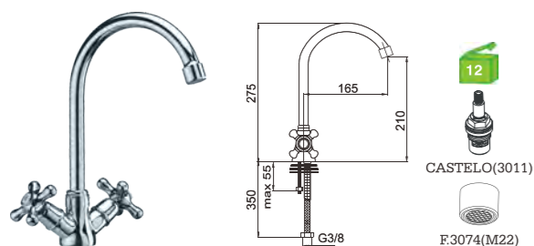
H15T5C Misturadora lava-loiça Kitchen mixer Monobloc fregadero BICA ---3068
