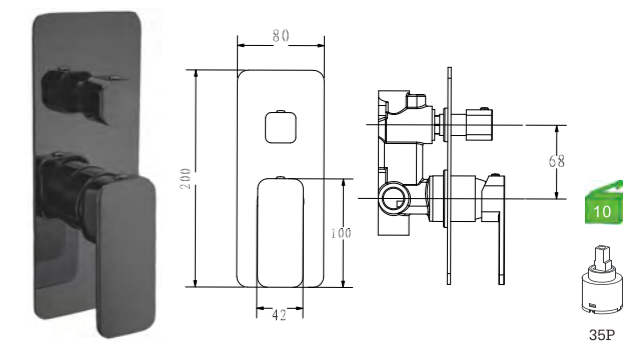
D21RP42BL(B) Monocomando embutido 2 vias Built-in mixer Monomando empotrado 2 vias
