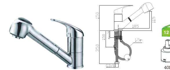
R26M7C C/Bicha Certificada Monocomando lava-loiça com chuveiro Kitchen mixer with pull out shower Monomando fregadero extraible C/CHUVEIRO---172 BICHA ---2028(1.5M)
