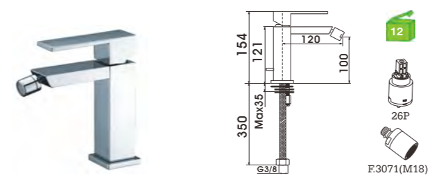
C51FT4C Monocomando bidé Bidet mixer Monomando bidet
