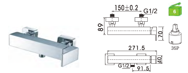
C51FX3C Monocomando duche Shower mixer Monomando ducha C/CHUVEIRO ---922 BICHA ---2030CR(1.7M) SUPORTE ---KH
