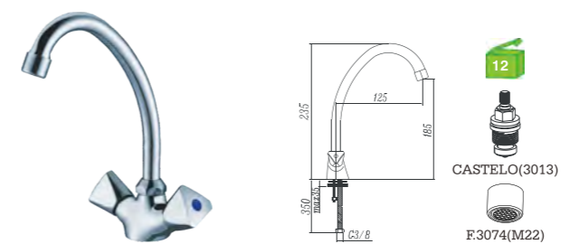
H11035C Misturadora lava-loiça Kitchen mixer Monobloc fregadero BICA ---3062
