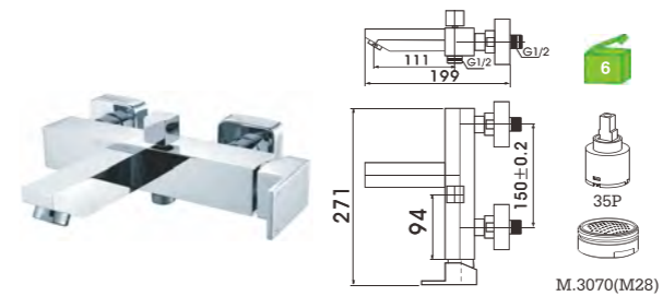
C53FX2C Monocomando banheira Bath/shower mixer Monomando baño C/CHUVEIRO---925 BICHA ---2031(1.7M) SUPORTE ---KH INVERSOR ---3035
