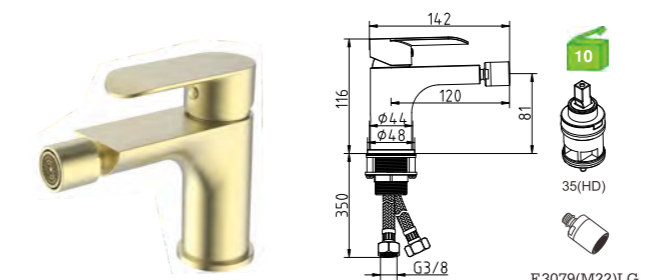
A60UP4LG Monocomando bidé Bidet mixer Monomando bidet
