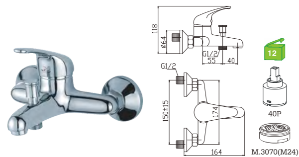
A68M2C Monocomando banheira Bath/shower mixer Monomando baño C/CHUVEIRO---168 BICHA ---2031(1.7M) SUPORTE ---JH INVERSOR ---3030
