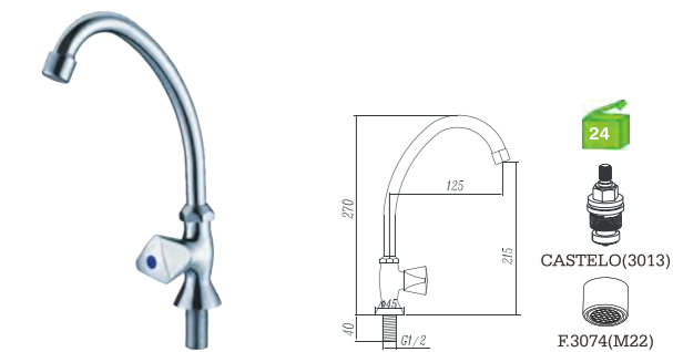
H11038C Torneira de balcão 1 água Kitchen faucet Grifo vertical 1 agua BICA ---3062
