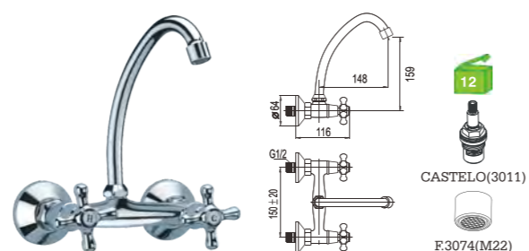
H15T9C Misturadora lava-loiça à parede bica alta Wall mouted kitchen mixer Monobloc fregadero pared (caño alto) BICA ---3062
