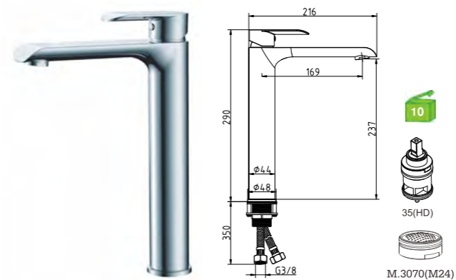
A60UP1C Monocomando lavatório alto Basin mixer Monomando lavabo alto C/bicha certificada S/VÁLVULA
