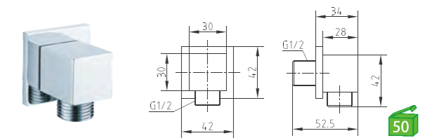
3091 Tomada de água Toma de água
