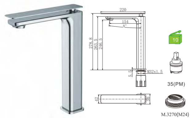
D22HK1C Monocomando lavatório alto Basin mixer Monomando lavabo alto
