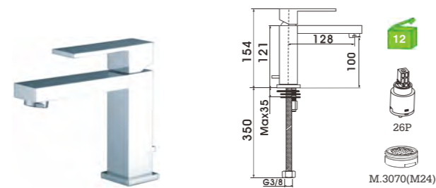
C51FT1C-1 Monocomando lavatório Basin mixer Monomando lavabo
