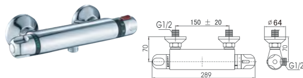
H14W3C Termostática – duche Thermostatic shower mixer Mezclador termostático ducha C/CHUVEIRO---918 BICHA ---2030CR(1.7M) SUPORTE ---JH
