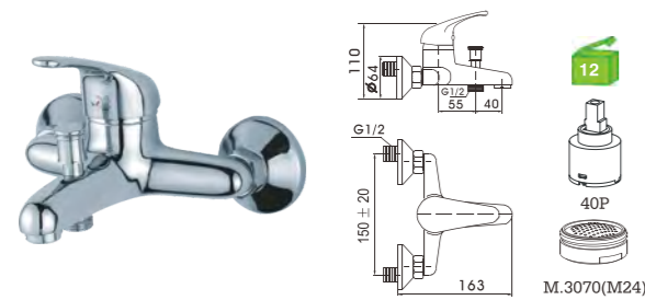
R26M2C C/CHUVEIRO---168 Monocomando banheira Bath/shower mixer Monomando baño C/CHUVEIRO---168 BICHA ---2031(1.7M) SUPORTE ---JH INVERSOR ---3030
