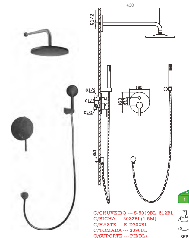
D26FK47BL Conj.Monocomando embutido 2 vias para duche Built-in shower mixer Conj.Monomando empotrado 2 vias para ducha
