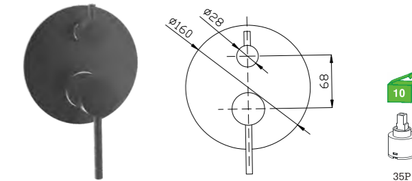
D26FK42BL(B) Monocomando embutido 2 vias Built-in mixer Monomando empotrado 2 vias
