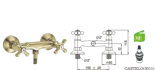
H15T3BR Misturadora ducha Shower mixer Monobloc ducha C/CHUVEIRO---888BR BICHA ---2030BR(1.7M) SUPORTE ---MH(BR)
