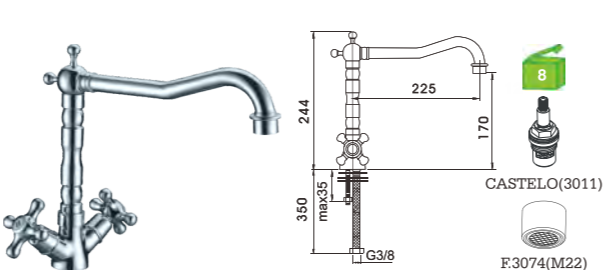
H15T15C Misturadora lava-loiça Kitchen mixer Monobloc fregadero
