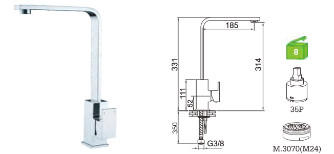
C51FX8C Monocomando lava-loiça Kitchen mixer Monomando fregadero
