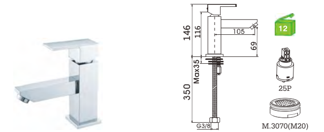
C53FD1C-1 Monocomando lavatório Basin mixer Monomando lavabo
