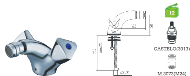
H11034C Misturadora bidé Bidet mixer Monobloc bidet
