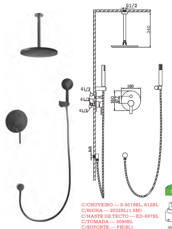
D26FK46BL Conj.Monocomando embutido 2 vias para duche Built-in shower mixer Conj.Monomando empotrado 2 vias para ducha
