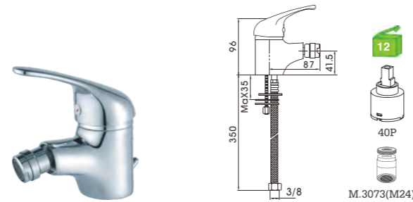
R26M4C C/Bicha Certificada Monocomando bidé Bidet mixer Monomando bidet
