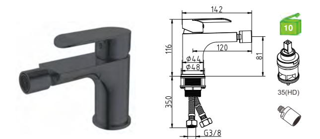
A60UP4BL Monocomando bidé Bidet mixer Monomando bidet
