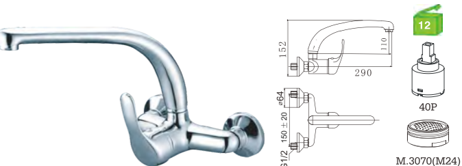
C17DF9C Monocomando lava-loiça à parede bica alta-fundida Wall mounted kitchen mixer Monomando fregadero pared (caño fundido)
