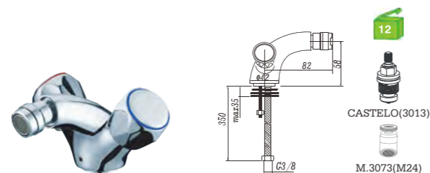
H11024C Misturadora bidé Bidet mixer Monobloc bidet
