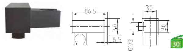
3093BL Tomada de água com suporte Toma de água com suporte
