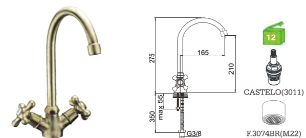
H15T5BR Misturadora lava-loiça Kitchen mixer Monobloc fregadero BICA ---3068(BR)
