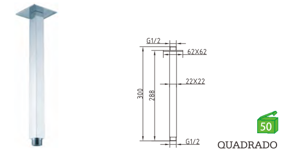
ED-696 Haste de tecto Barra de tecto
