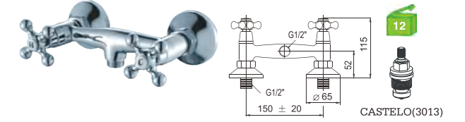
H11T3C Misturadora duche Shower mixer Monobloc ducha C/CHUVEIRO---168 BICHA ---2031(1.7M) SUPORTE ---JH
