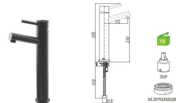
E34GP1BL Monocomando lavatório alto Basin mixer Monomando lavabo alto C/bicha certificada S/VÁLVULA
