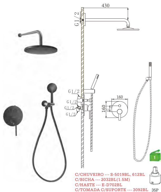
D26FK44BL Conj.Monocomando embutido 2 vias para duche Built-in shower mixer Conj.Monomando empotrado 2 vias para ducha
