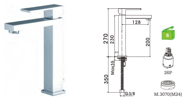
C51FT1C Monocomando lavatório alto Basin mixer Monomando lavabo alto
