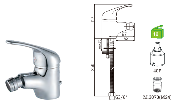
A68M4C Monocomando bidé Bidet mixer Monomando bidet
