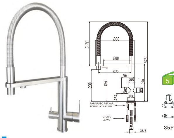
H30LP8X C/bicha certificada Monocomando lava-loiça dupla função da água purificada industrial Kitchen mixer double function – purified water Monomando fregadero doble función – agua Ósmosis industrial
