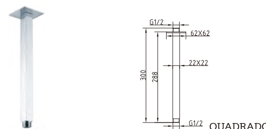
ED-696 Haste de tecto Barra de techo
