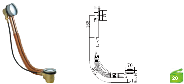
A203 Válvula automática para banheira
