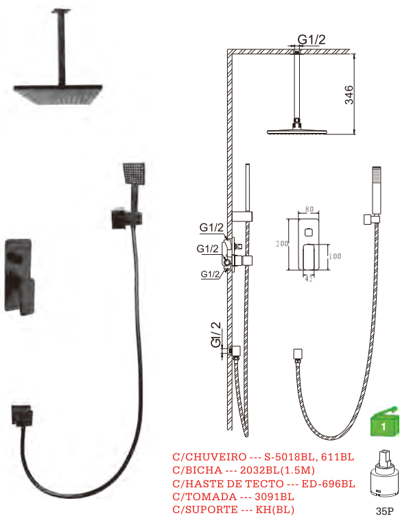
D21RP45BL Conj.Monocomando embutido 2 vias para duche Built-in shower mixer Conj.Monomando empotrado 2 vias para ducha
