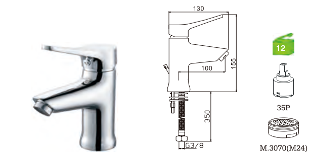
C38DA1C Monocomando lavatório Basin mixer Monomando lavabo
