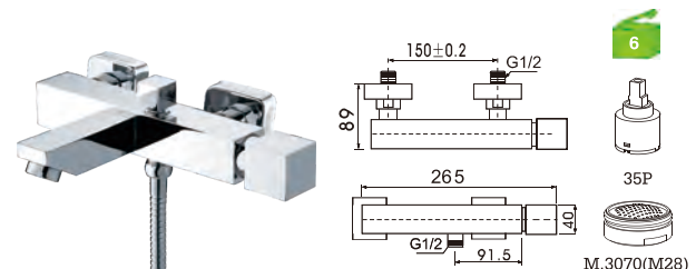
C50EB2C Monocomando banheira
