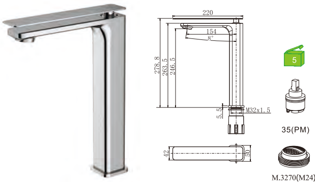
D22HK1C Monocomando lavatório alto Basin mixer Monomando lavabo alto
