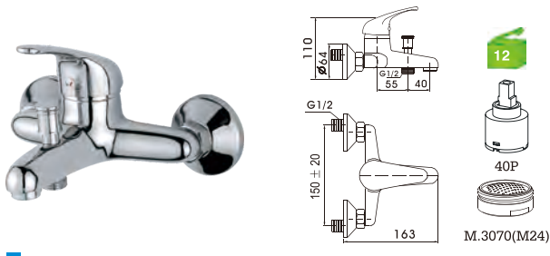
R26M2C Monocomando banheira Bath/shower mixer Monomando baño C/CHUVEIRO---168 BICHA ---2031(1.7M) SUPORTE ---JH INVERSOR ---3030
