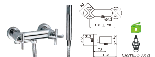
C30X3C Misturadora duche Shower mixer Monobloc ducha C/CHUVEIRO---918 BICHA ---2030CR(1.7M) SUPORTE ---TH
