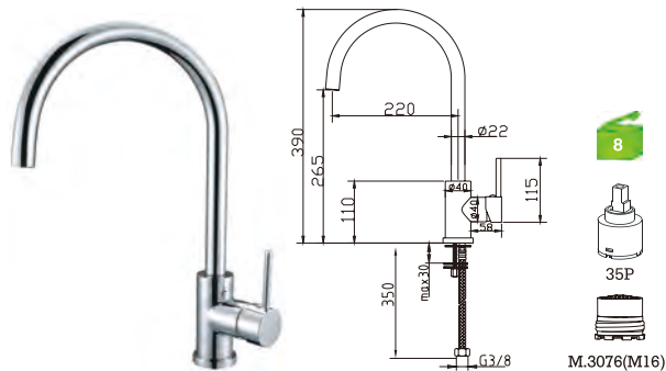
E37GB5C Monocomando de lava-loiça Kitchen mixer Monomando de fregadero
