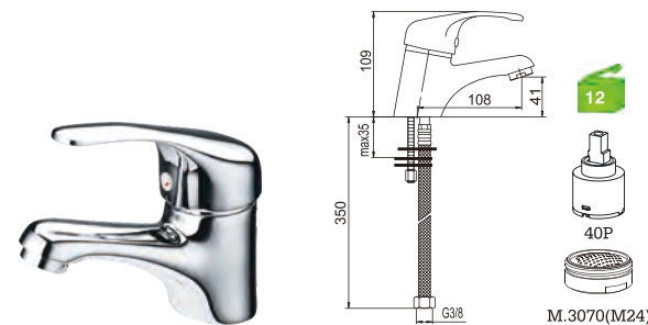
C15DF1C Monocomando lavatório Basin mixer Monomando lavabo
