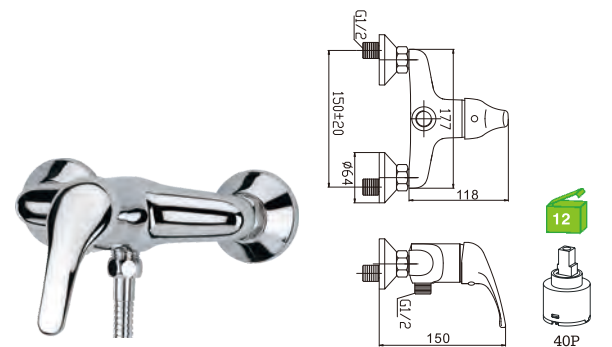
A68M3C Monocomando duche Shower mixer Monomando ducha C/CHUVEIRO---168 BICHA ---2031(1.7M) SUPORTE ---JH
