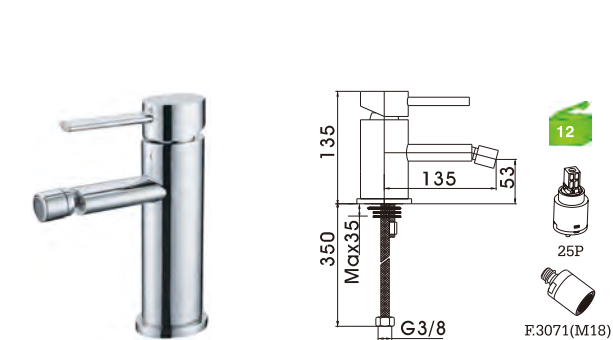
C62GD4C Monocomando bidé Bidet mixer Monomando bidet
