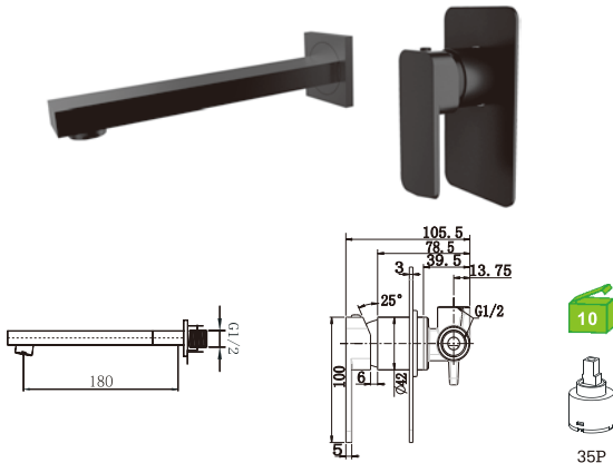
D21RP10BL Monocomando lavatório embutido In wall basin mixer Monomando lavabo empotrado
