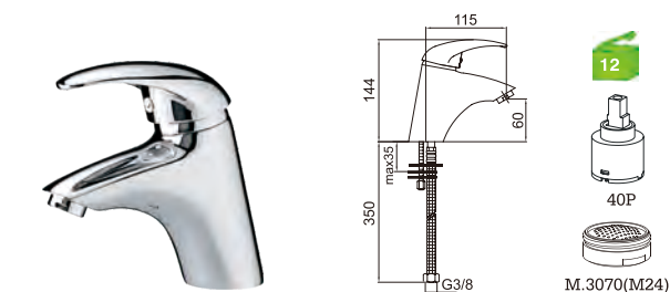
C21N1C Monocomando lavatório Basin mixer Monomando lavabo
