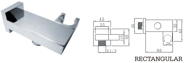
3094 Toma de água com suporte Toma de agua con soporte
