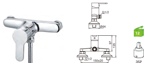
C08GS3C Monocomando duche Shower mixer Monomando ducha C/CHUVEIRO ---168 BICHA ---2031(1.7M) SUPORTE ---JH
