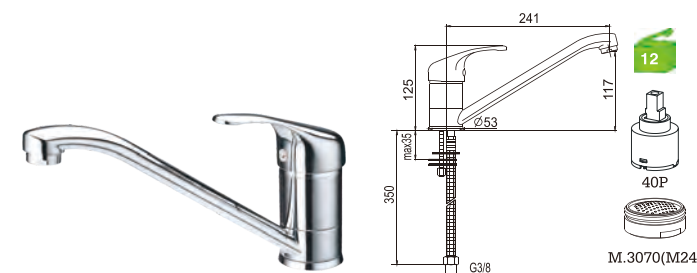
C15DF5C Monocomando lava-loiça Kitchen mixer Monomando fregadero (caño bajo)
