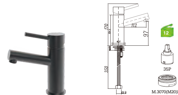
E34GP1BL-1 Monocomando lavatório Basin mixer Monomando lavabo
