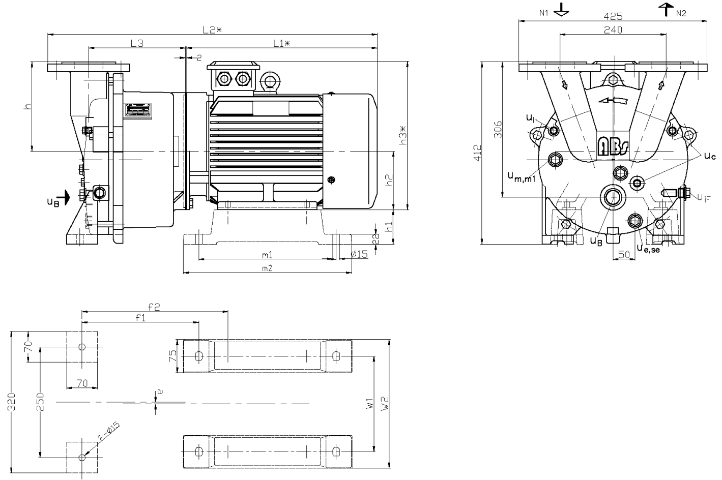
外形尺寸 VA 325, VA 425
