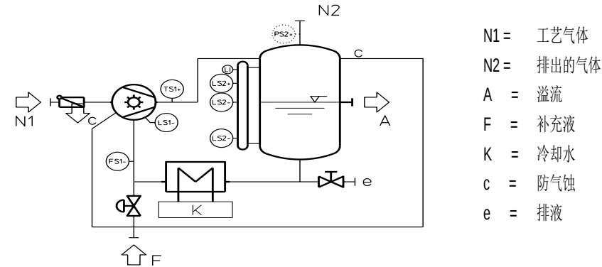
流程图: 带选择性安全装置的真空泵系统
