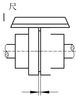
图 5.C.2 对中检查
