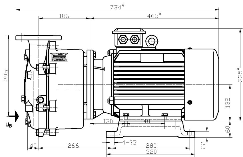
外形尺寸 VA 250
