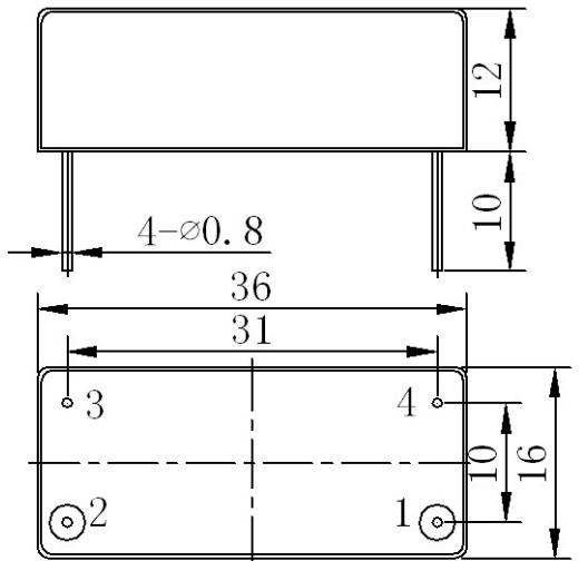
Bottom View Unit:mm
