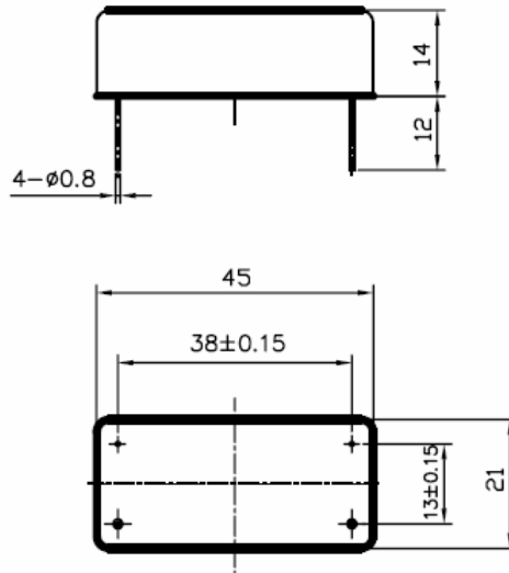
封装结构图
