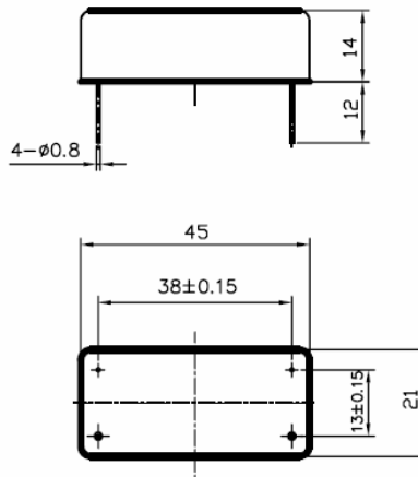
封装结构图
