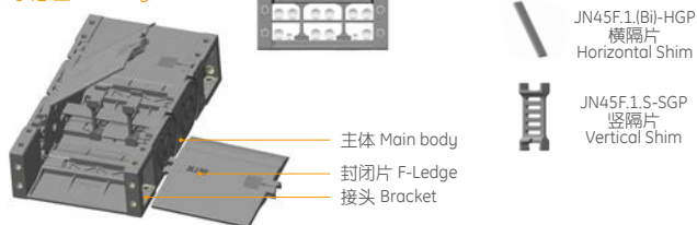
示意图 Drawing
