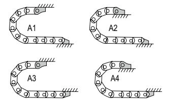
斜接头安装方式 Connector mounting way
