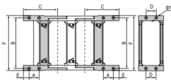
F-Q 型接头 F-Q type bracket
