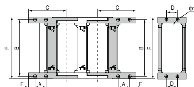
F-O 型接头 F-O type bracket
