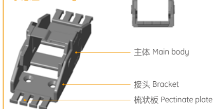
示意图 Drawing
