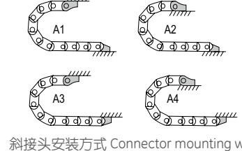
斜接头安装方式 Connector mounting way
