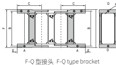
F-Q 型接头 F-Q type bracket
