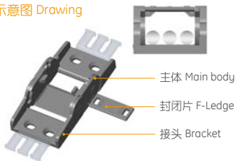
示意图 Drawing
