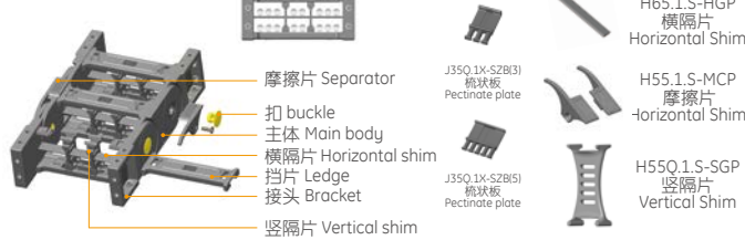
示意图 Drawing
