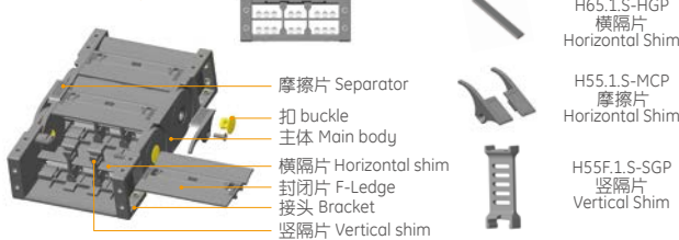
示意图 Drawing
