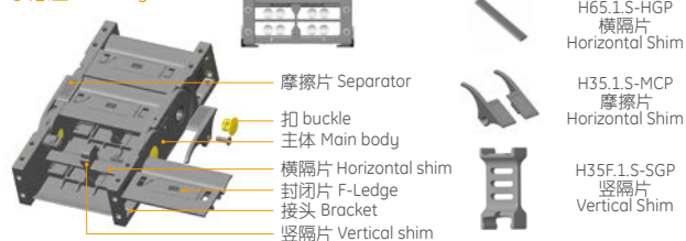
示意图 Drawing
