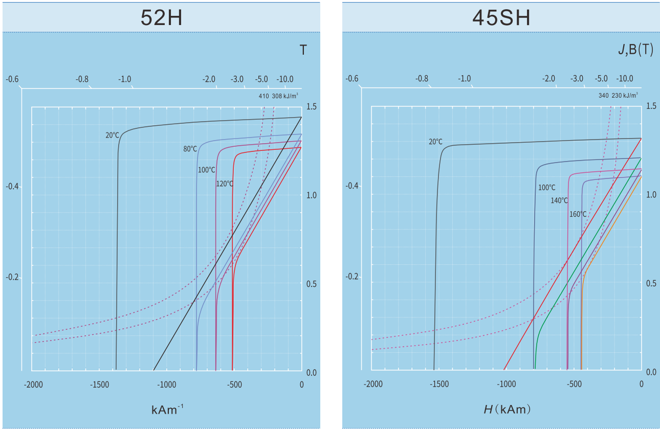
退磁曲线图 DEMAGNETIZATION CURVE
