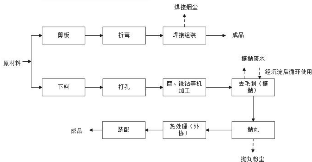
图 2.3-1 项目生产工艺流程及产污环节图
