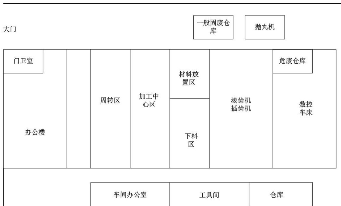
图 2.1-1 厂区总平面布置图
