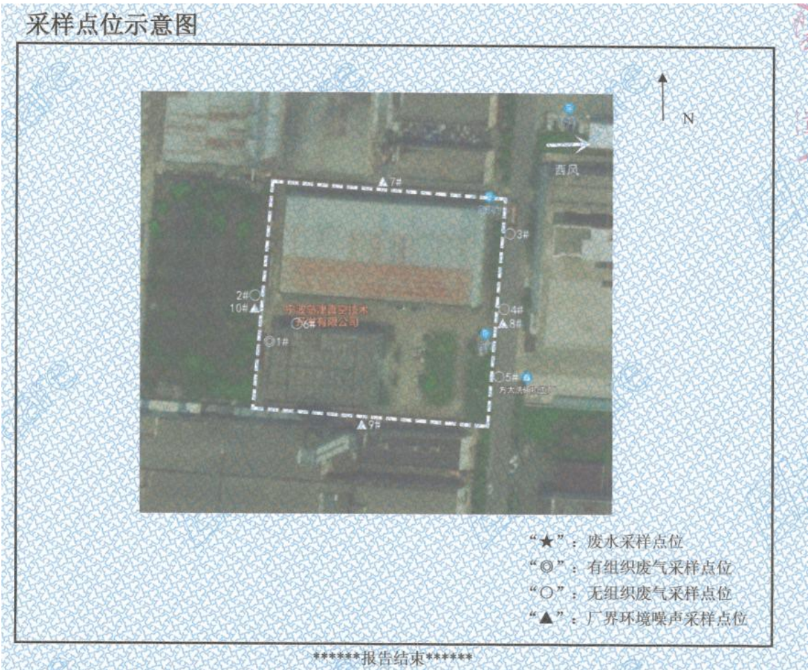
图 3.5-1 有、无组织废气、废水及厂界噪声检测布点图
