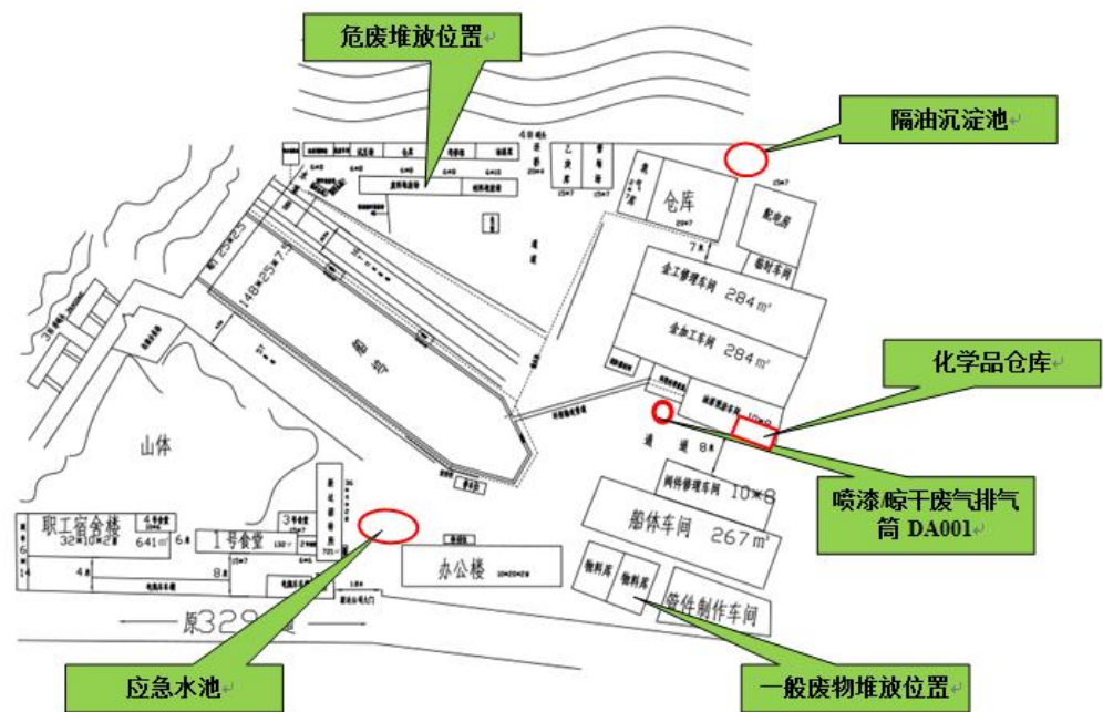
图 3-1 厂区布置平面图
