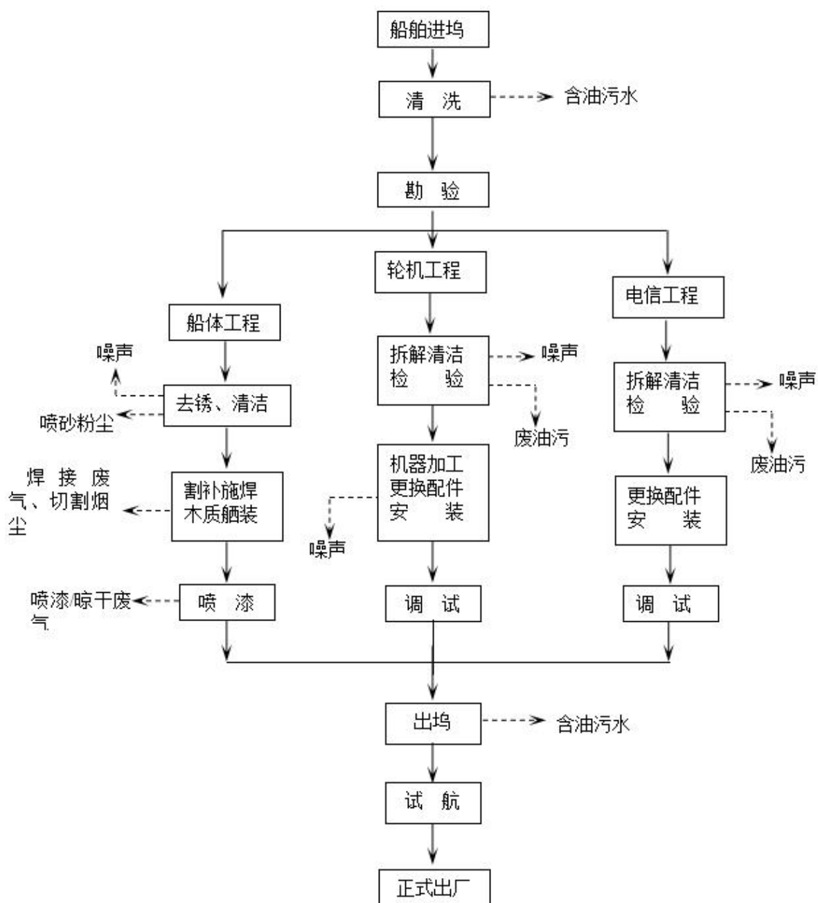
图 3-2 船舶维修工艺流程图
