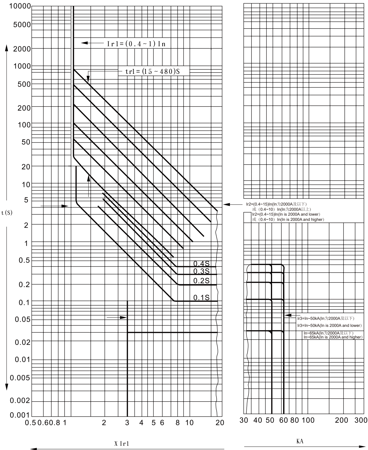
过电流控制器保护特性
