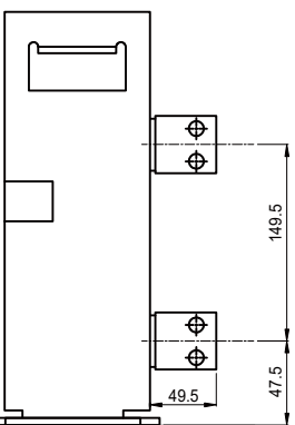
垂直接线 Vertical wiring
