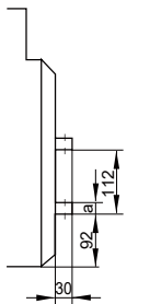
垂直接线 Vertical wiring
