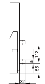
水平接线 Horizontal wiring
