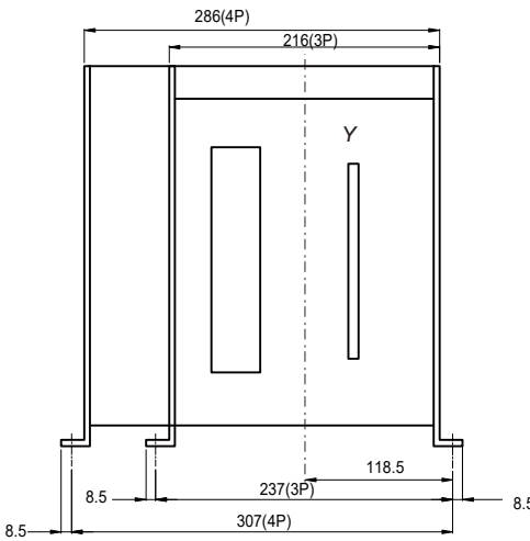
水平接线 Horizontal wiring
