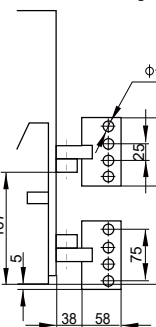
垂直接线 Vertical wiring
