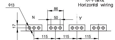
水平接线 Horizontal wiring
