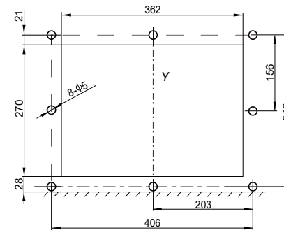
Y: 断路器面罩中心线 Circuit breaker mask center line
