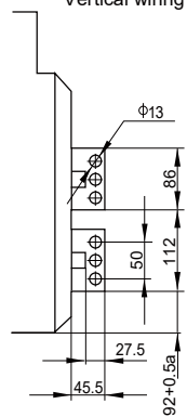
垂直接线 Vertical wiring
