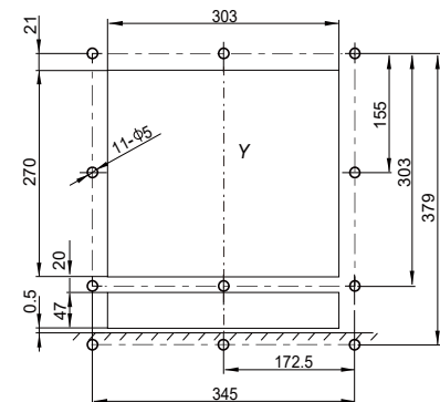
Y: 断路器面罩中心线 Circuit breaker mask center line
