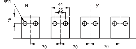
水平接线 Horizontal wiring
