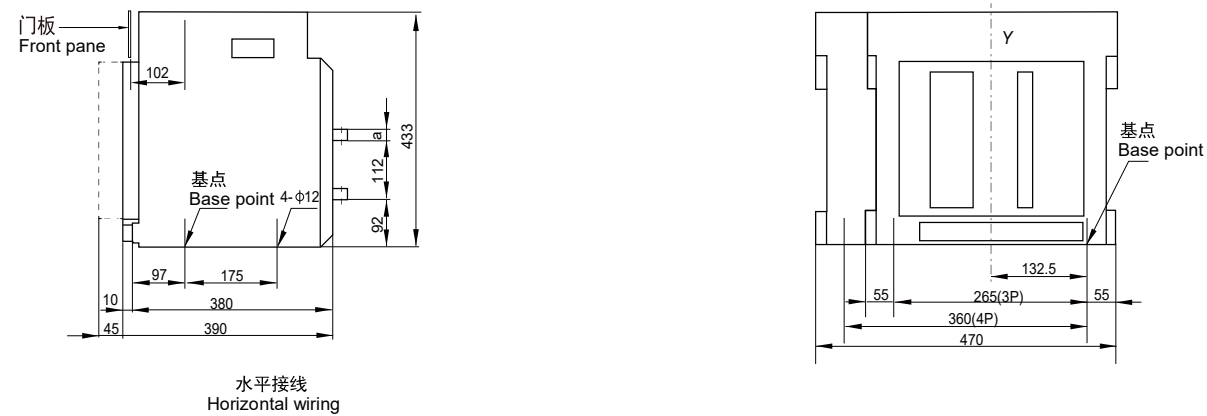
水平接线 Horizontal wiring
