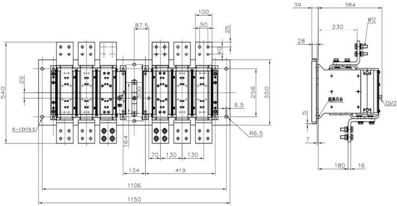
XKQFS 4000/3P 尺寸图:
