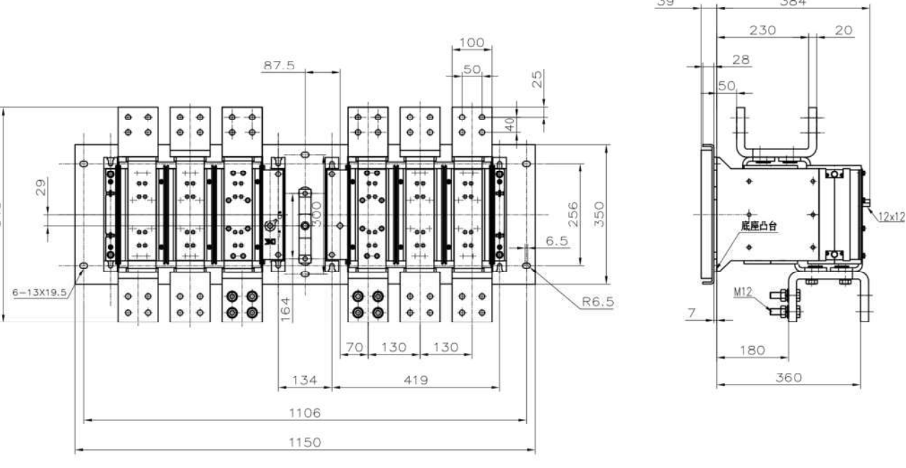
XKQFS 5000/3P 尺寸图:
