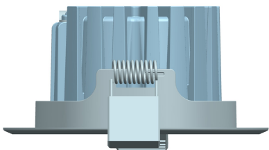
左视图
