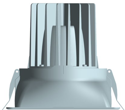
设计1主视图
